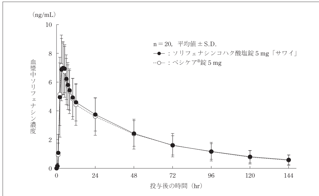
図1 血漿中ソリフェナシン濃度
