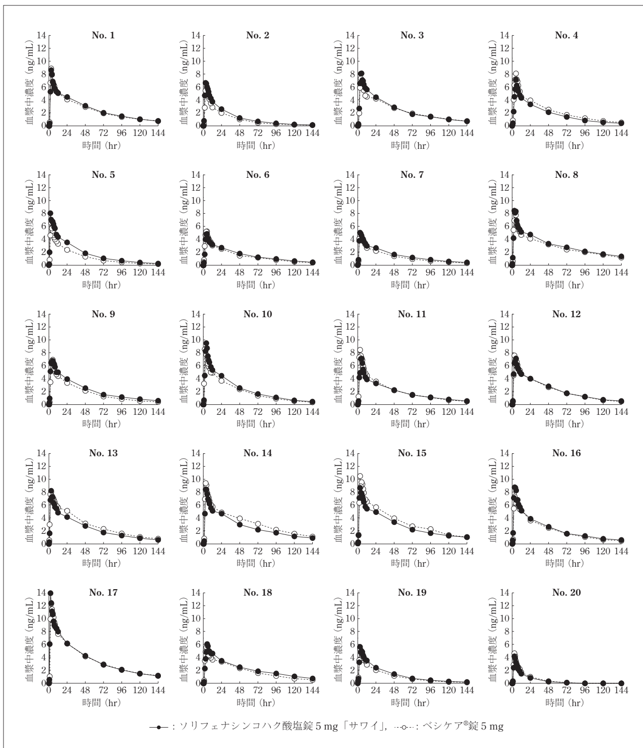
図2 各被験者の血漿中ソリフェナシン濃度
